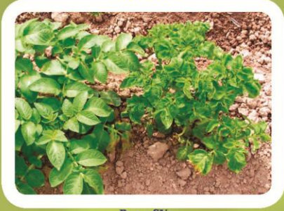
Вирус SY
